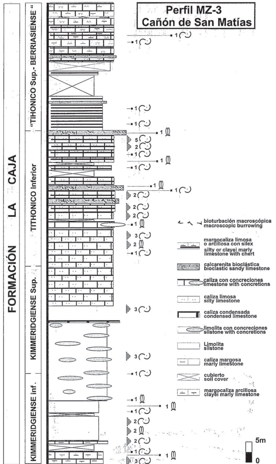
Fig. 2- Columna litológica sintética del perfil MZ-3 (Cañón de San Matías, Zacatecas). Posición estratigráfica aproximada de asociaciones de bivalvos, autóctonas (M) y alóctonas (C). Los números indican las asociaciones reconocidas en uno o en varios horizontes de registro de megabentos.
